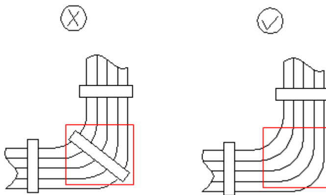
图4-22 线缆捆扎示意图（三）
