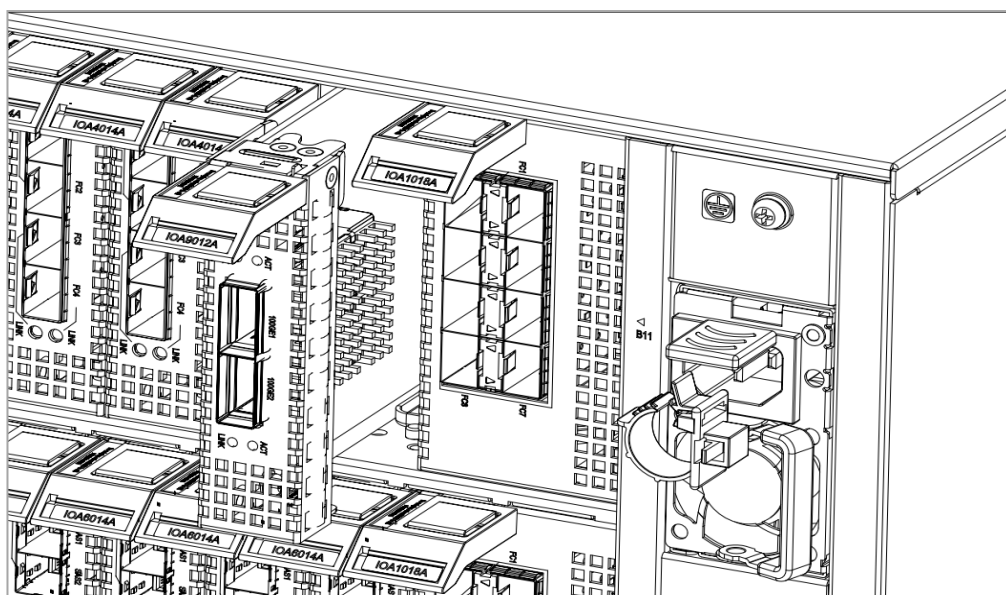
图6-9 安装/拆卸 IO 插卡示意图
