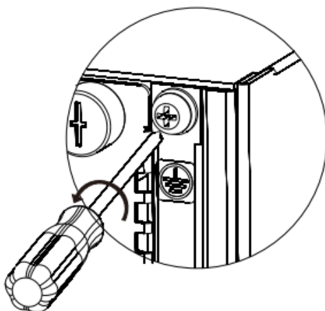
图4-25 松开设备接地端子的螺钉示意图
