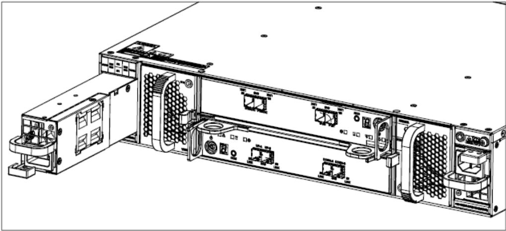
图6-8 安装/拆卸 SSU2225B 电源模块示意图
