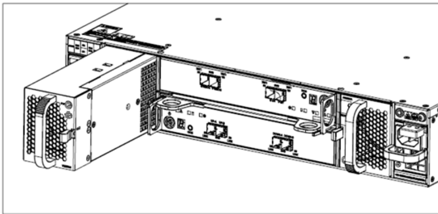
图6-6 安装/拆卸 SSU2225B 风扇模块（含电池模块）示意图
