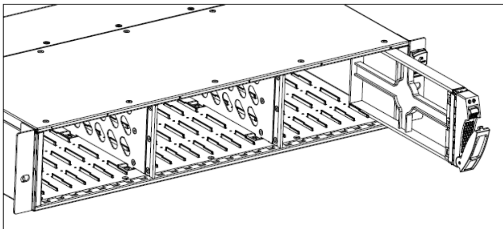
图6-14 安装 SSU 磁盘假面板示意图
