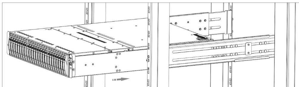
图4-18 安装 SSU2225 示意图
