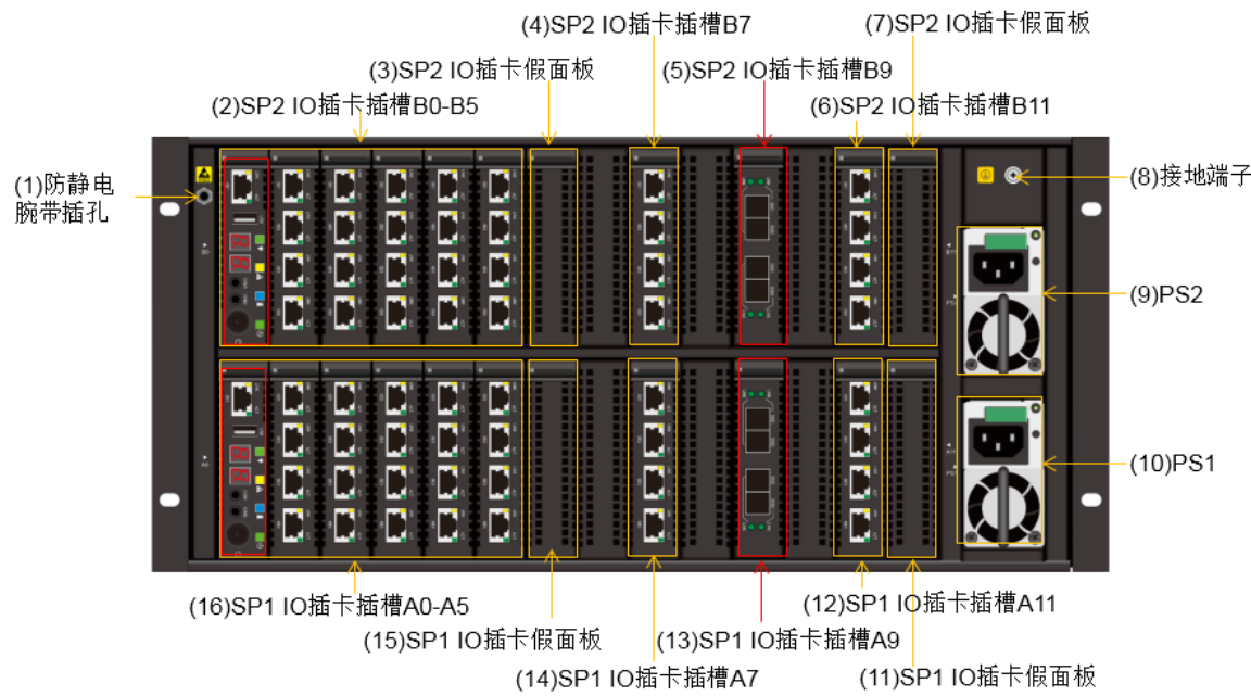
图3-2 SPU 后正视图
