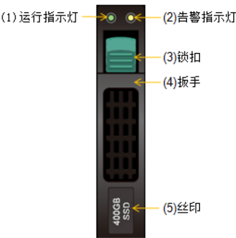
图3-15 SSU 磁盘模块前面板
