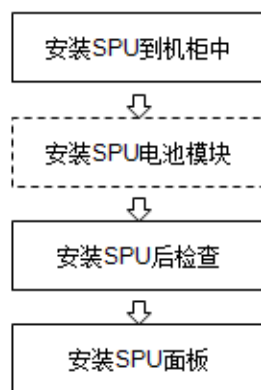
图4-11 SPU 安装流程示意图
