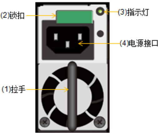
图3-7 SPU 电源模块正视图
