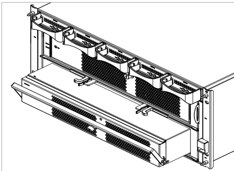
图6-4 安装/拆卸 SPU 风扇模块示意图
