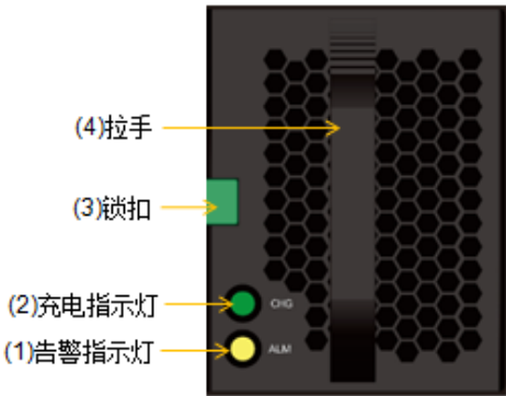
图3-12 SSU2225B 风扇模块（含电池模块）正视图
