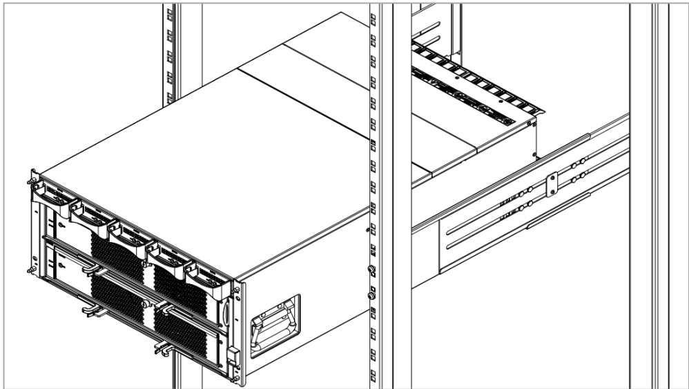
图4-12 安装 SPU 示意图
