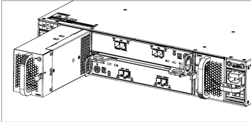
图6-7 安装/拆卸 SSU2225 风扇模块示意图
