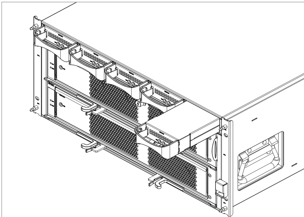
图4-13 安装 SPU 电池模块示意图
