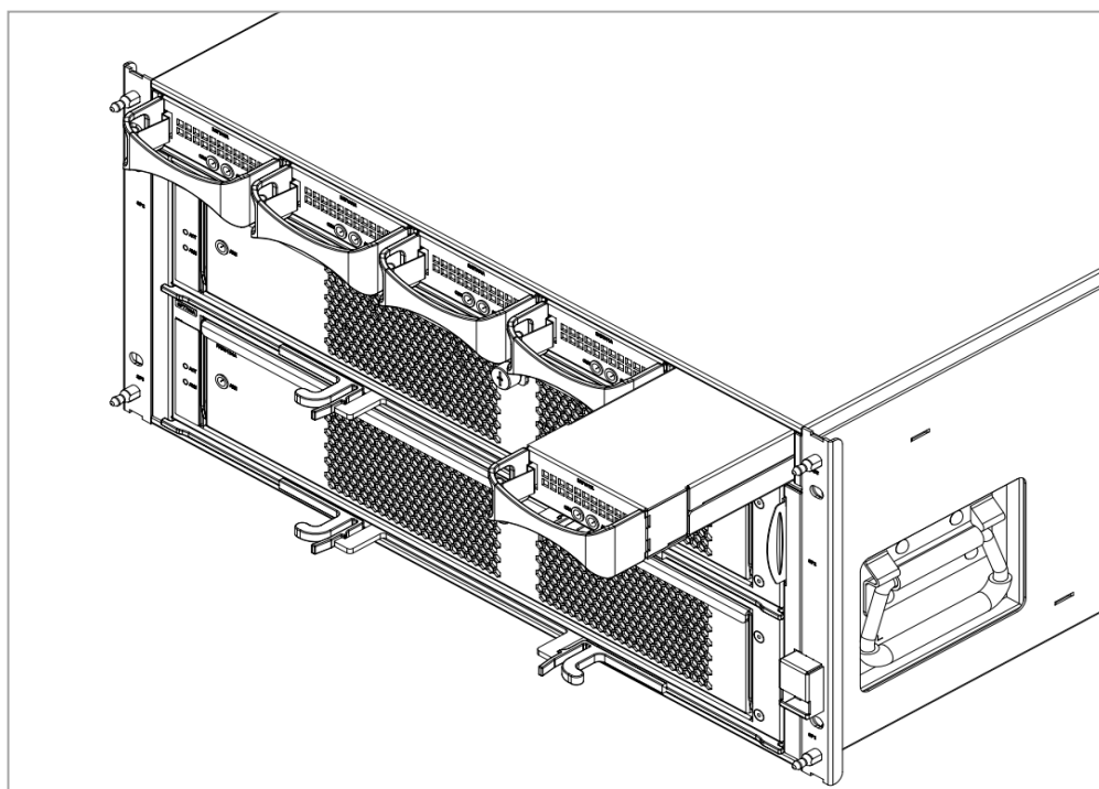
图6-5 安装/拆卸 SPU 电池模块示意图
