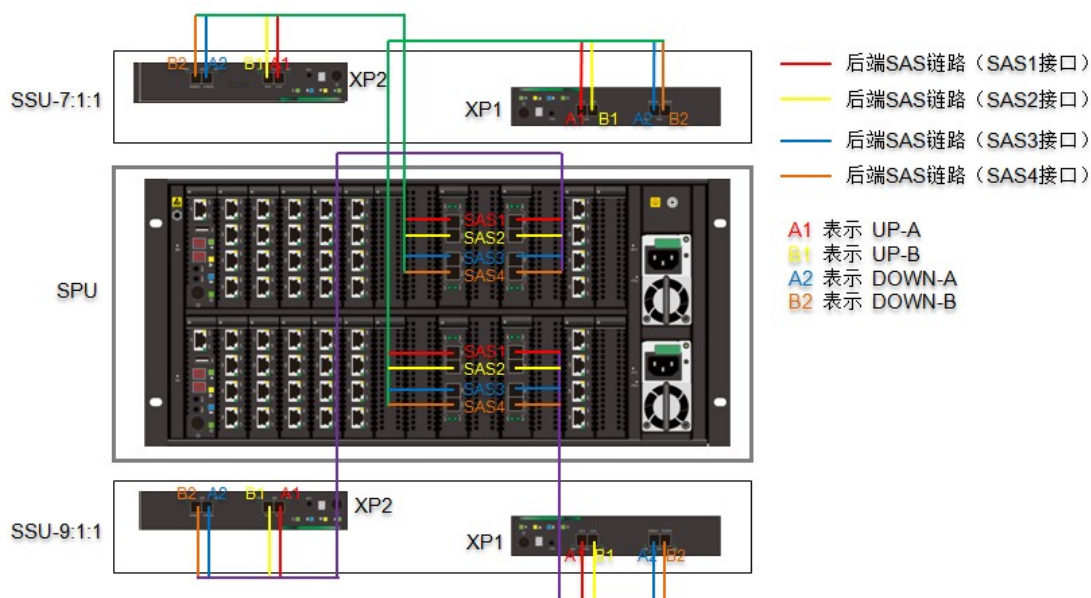
图4-35 SAS 线缆安装示意图
