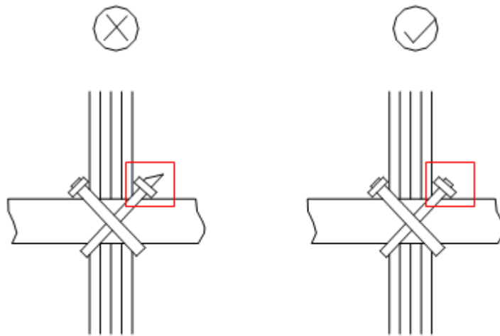
图4-21 线缆捆扎示意图（二）
