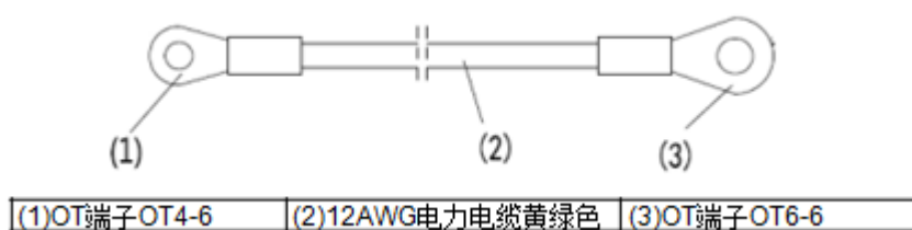
图4-24 接地线示意图
