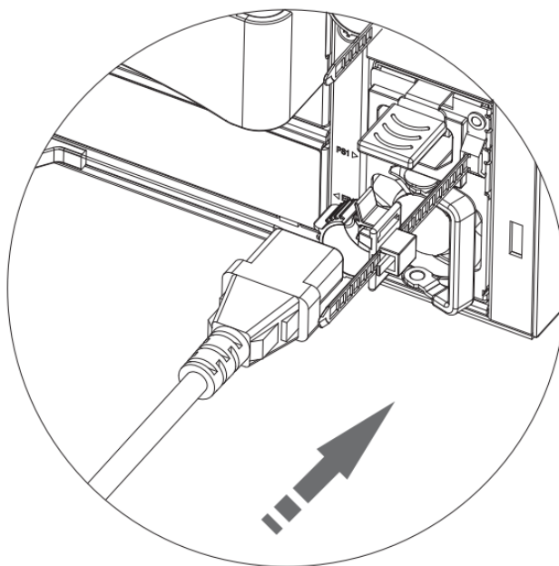
图4-28 安装电源线示意图（一）
