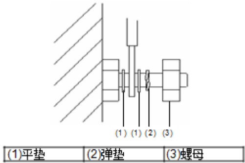
图4-19 固定线缆端子示意图
