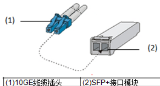
图4-39 10GE 线缆和接口示意图
