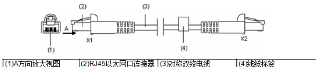
图4-38 GE 线缆示意图
