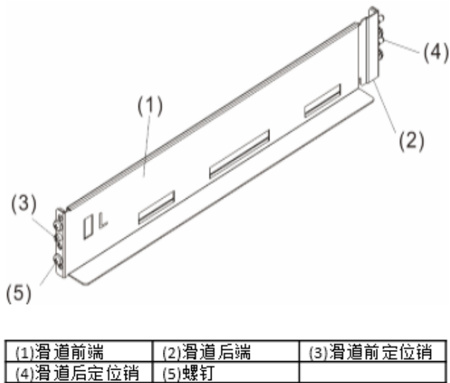
图4-6 带定位销托架式滑道（左侧滑道）示意图
