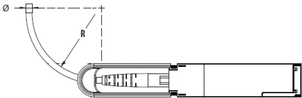
图4-34 AOC 光缆弯曲半径示意图
