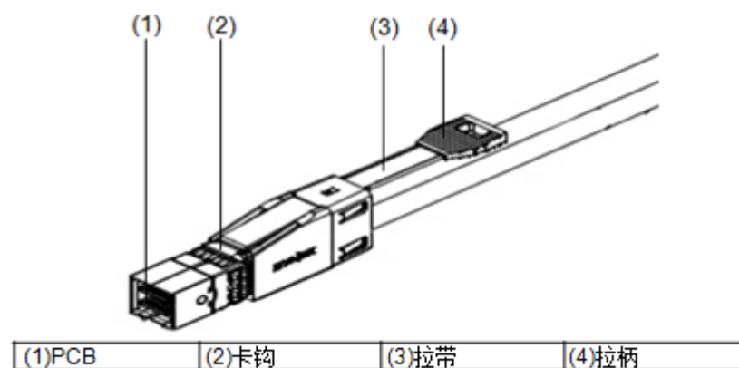
图4-32 SAS 线缆上 Mini SAS HD 连接器示意图
