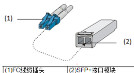
图4-37 FC 线缆和接口示意图
