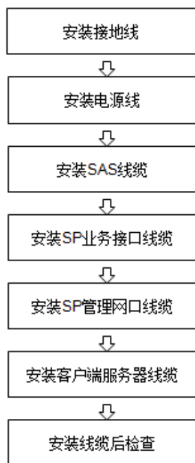
图4-23 线缆安装流程示意图
