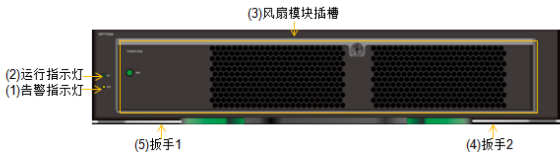
图3-3 SP 正视图
