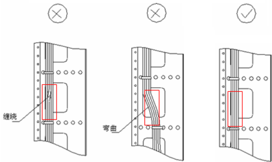
图4-20 线缆捆扎示意图（一）
